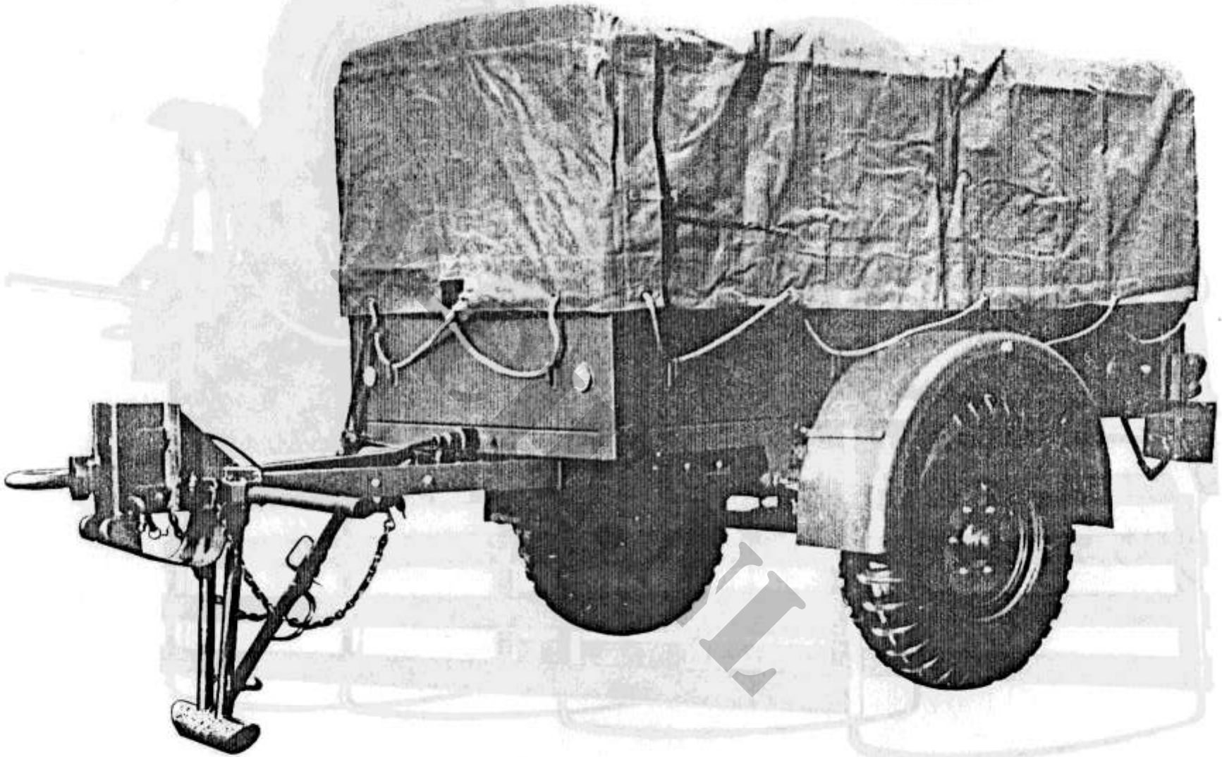
VOORAANZICHT VOERTUIG
