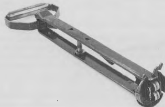
Figuur 22 Leg- en tordeerapparaat
