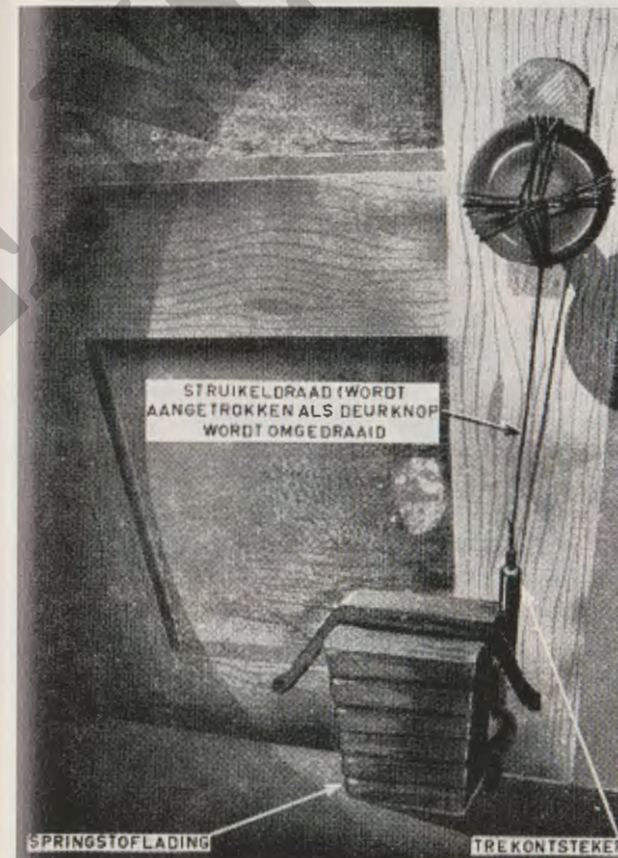
Fig. 16-14 Gevalstrikte deur
