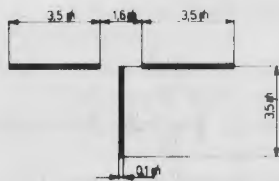
Figuur 17 Richtmerk
