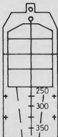
Figuur 12 Het mondvizier Model M 72 A 2
