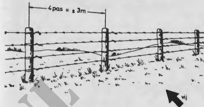
Figuur 9 4-draads afrastering
