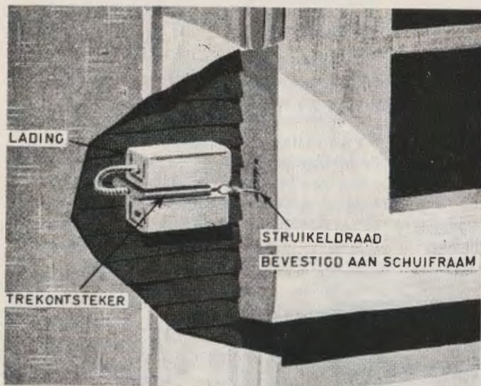
Fig. 16-15 Valstrik aan schuifraam
