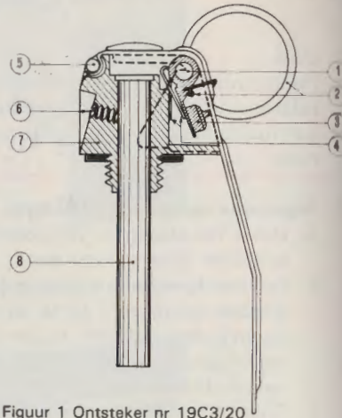
Figuur 1 Ontsteker nr 19C3/20
