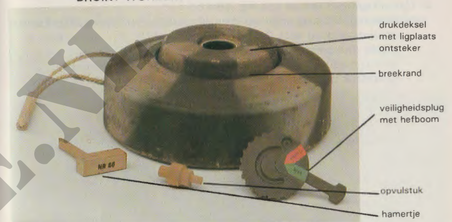
Fig. 16-2 Controle Trotylmijn AT nr. 26C1
