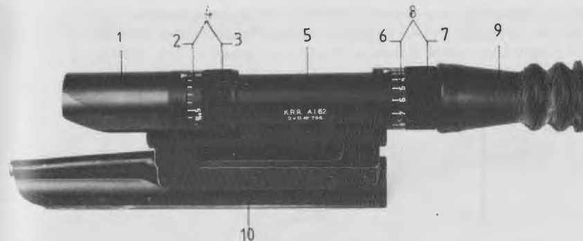
Figuur 18 Richtkijker
