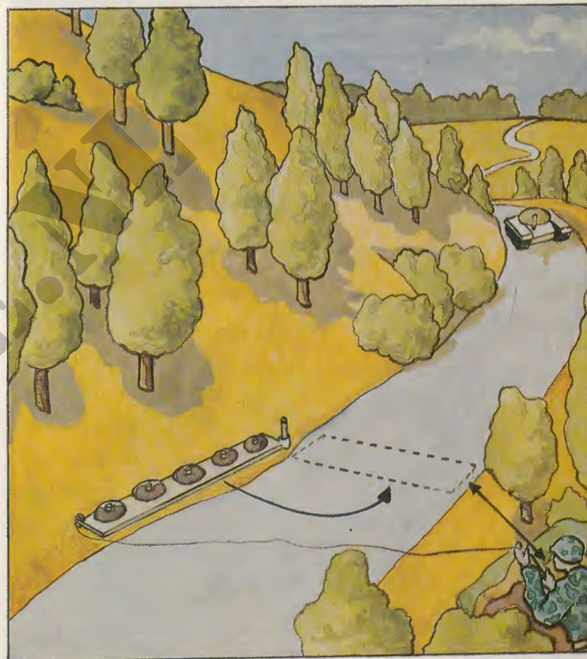
Figuur 10 Mijnenplank: 4-6 scherpgestelde AT-mijnen op een plank gebonden, onderlinge afstand max. 60 cm N.B. afstand bedienaar – plank/ketting min. 25 m
